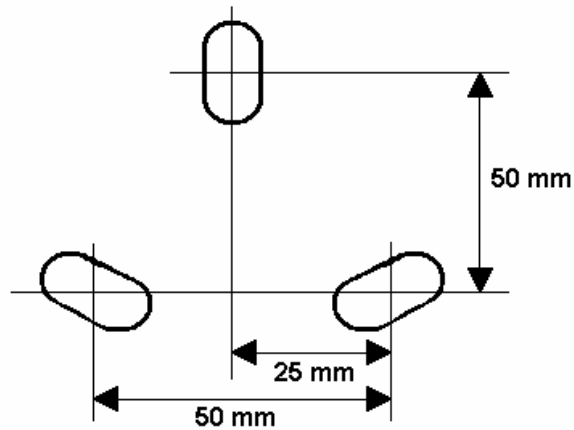
3 x Langloch 13 x 5 mm
